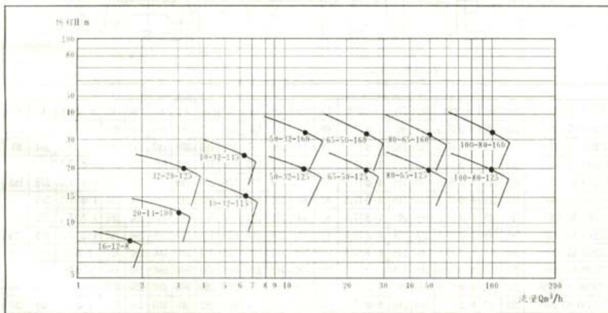
CQB型氟塑料磁力泵谱图
